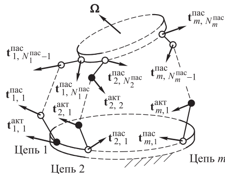
Рис. 2. Единичные кинематические винты обобщенного механизма параллельной структуры
